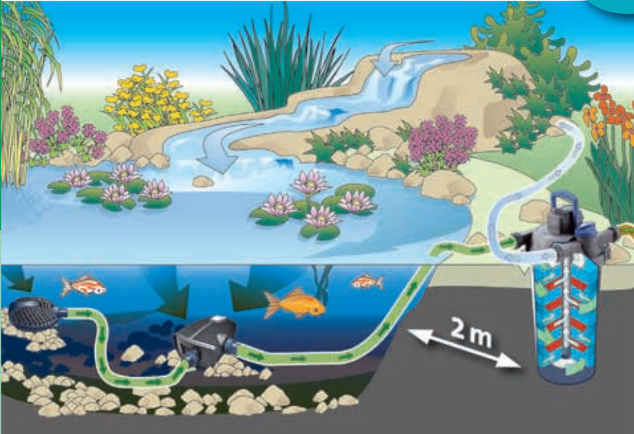
Représentation schématique : Filtre sous pression FiltoClear en combinaison avec pompe pour filtre et ruisseau
